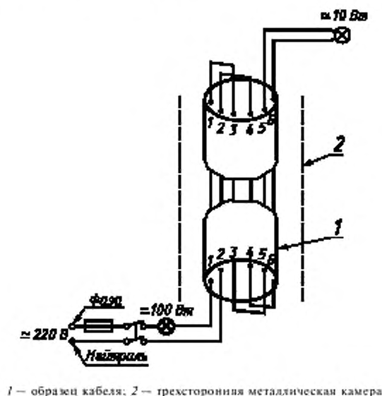
Рисунок 6 — Электрическая схема для испытания на нераспространение горения
