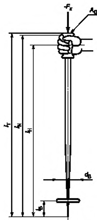
Рисунок 2 — Условное обозначение размеров горнолыжной палки
