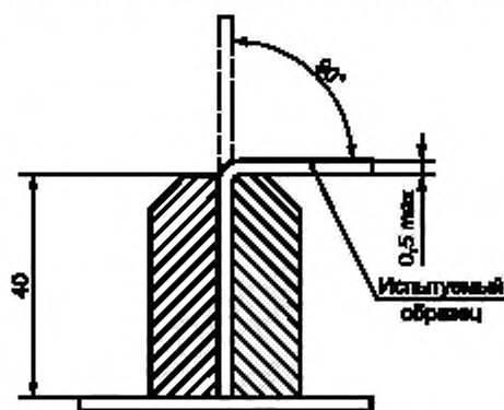
Рисунок 2 — Перегибание образца
