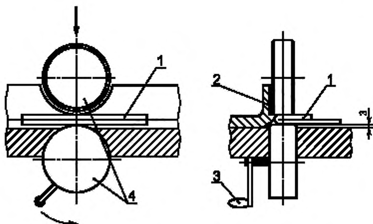
1 — испытуемый образец, 2 — стопор, 3 — рукоятка, 4 — валики
