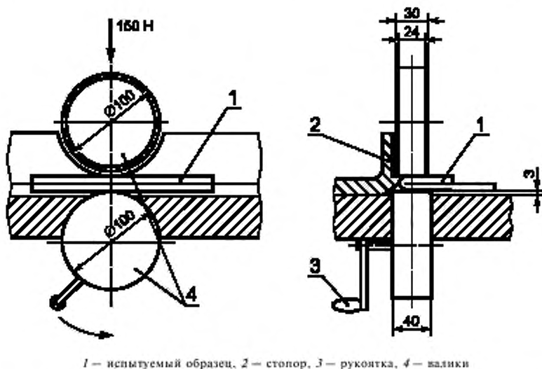
Рисунок 1 — Приспособление для прокатки места перегиба образцов материала
