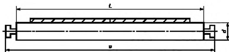
Рисунок 5 — Однораликовая опора
