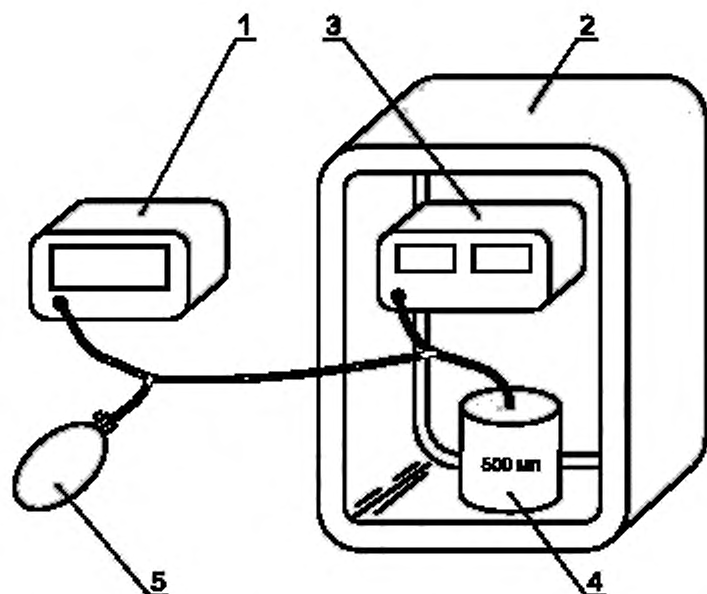
1 — эталонный манометр [8.1.1, перечисление б)]; 2 — климатическая камера [8.2.1, перечисление б)]; 3 — манометр испытываемого устройства; 4 — металлический сосуд [8.1.1, перечисление а)]; 5 — нагнетатель давления [8.1.1, перечисление с)]
