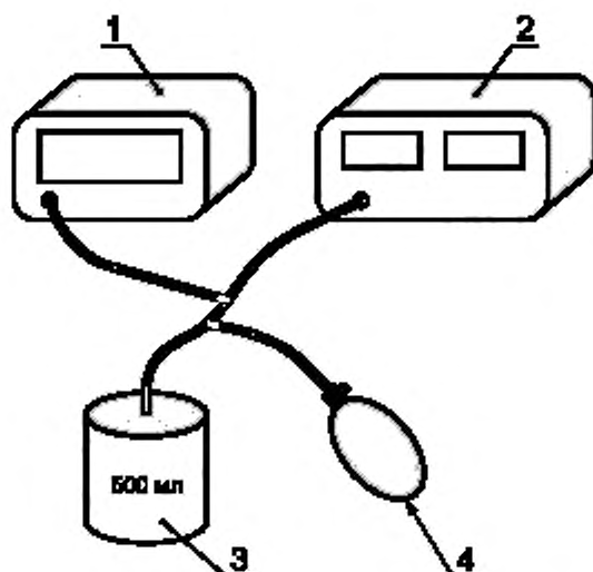
1 — эталонный манометр [8.1.1, перечисление б)]; 2 — манометр испытываемого устройства; 3 — металлический сосуд [8.1.1, перечисление а)]; 4 — нагнетатель давления [8.1.1, перечисление с)]
