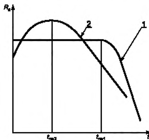
Рисунок 3 — Определение времени проникновения t_{пр} агрессивных сред по различным видам записываемых потенциометром кривых изменения во времени поверхностного электрического сопротивления R_s
