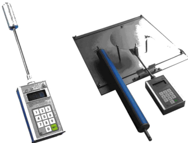
Рисунок 1 — Прибор для измерения напряженности электростатического поля СТ-01
