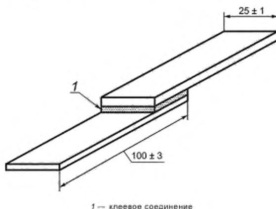
Рисунок 1 — Соединение внахлест
