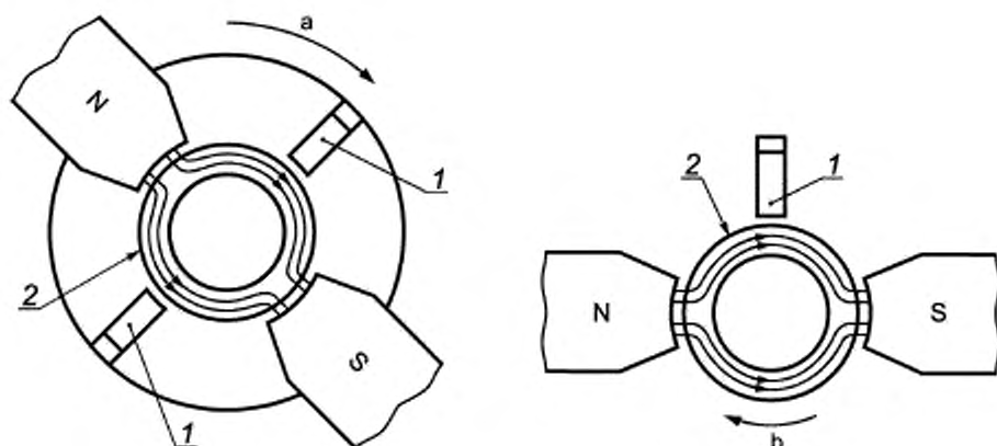
1 — преобразователь магнитного потока, 2 — труба; N — северный полюс; S — южный полюс
