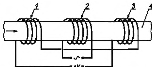
1 — вторичная катушка 1; 2 — первичная катушка; 3 — вторичная катушка 2; 4 — труба;
