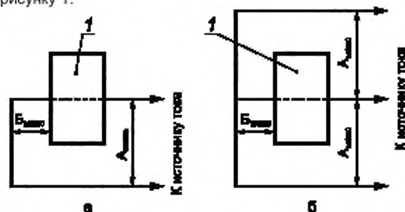
1 — испытываемый трансформатор, A_{\max} — расстояние между осями проводников соседних фаз в месте установки трансформатора в эксплуатации; B_{\max} — расстояние в свету от трансформатора до места ближайшего изгиба проводника, служащего в эксплуатации первичной обмоткой трансформатора
