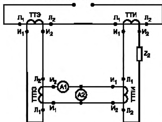
ТТЭ — эталонный трансформатор тока; ТТИ — испытуемый трансформатор тока; ТТПИ — промежуточный трансформатор тока, находящийся в цепи испытуемого трансформатора тока; ТТПЭ — промежуточный трансформатор тока, находящийся в цепи эталонного трансформатора тока. А1, А2 — амперметры; Z_2 — вторичная нагрузка в цепи испытуемого трансформатора тока
