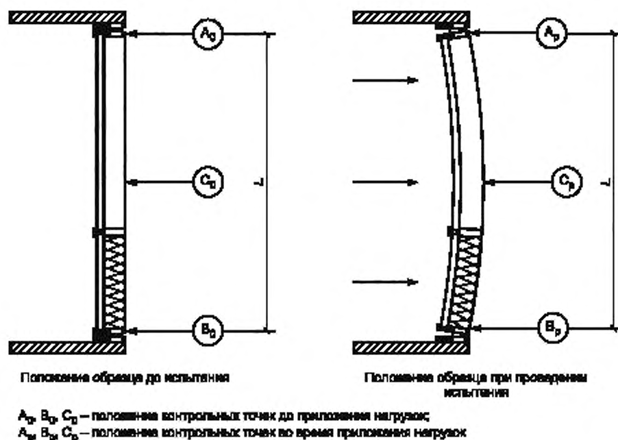
Рисунок А.1 — Схема установки измерительных приборов
