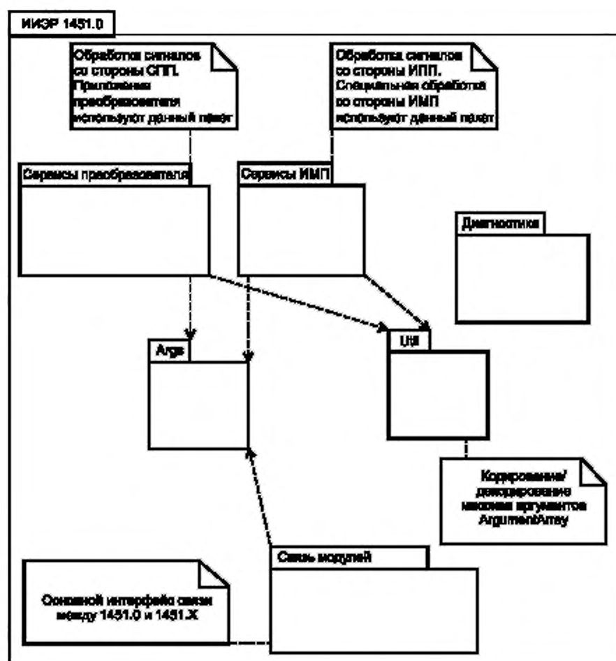
Рисунок 21 — Структура API
