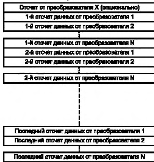
Рисунок 6 — Методы комбинирования наборов данных
