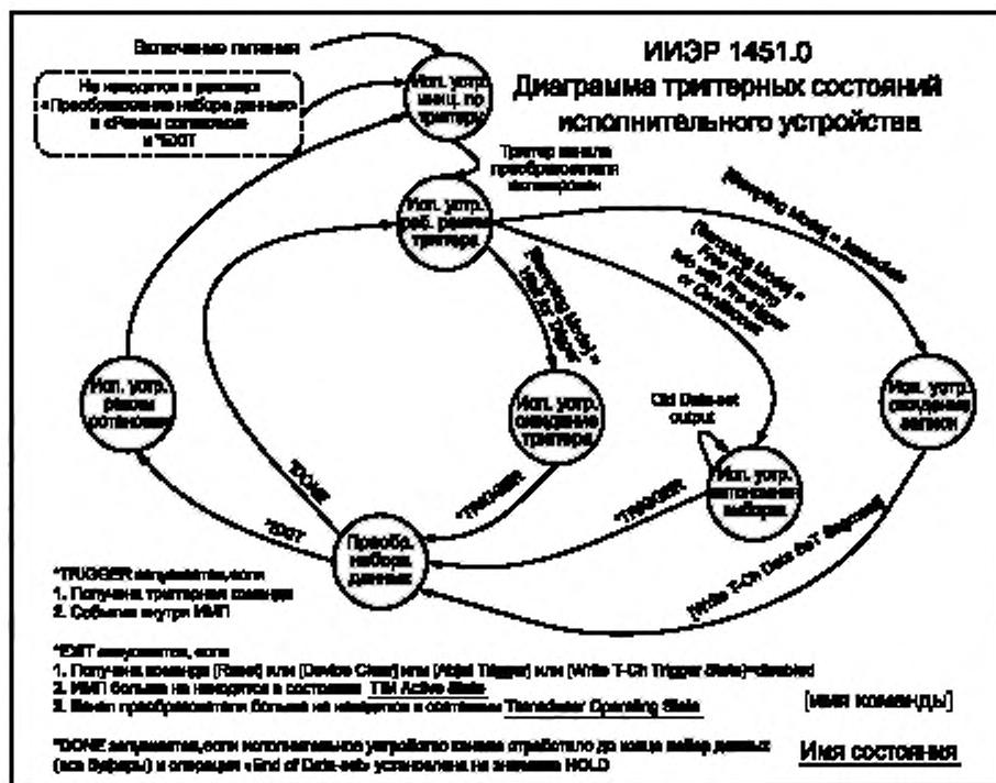
Рисунок 8 — Триггерные состояния исполнительного устройства
