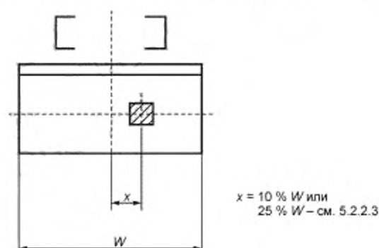
Рисунок 1 – Номинальная грузоподъемность при смещении от центра
