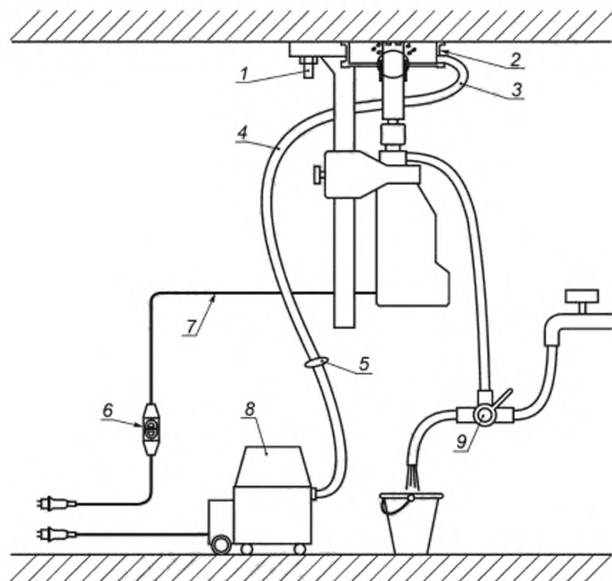
1 — сверлильная стойка с креплением анкерами; 2 — устройство для сбора жидкости; 3 — соединение с приспособлением для откачки жидкости; 4 — шланг для отвода жидкости; 5 — насадка пылесоса для «мокрого» сверления; 6 — УЗО (устройство защитного отключения), если поставляется; 7 — шнур питания; 8 — пылесос для «мокрого» сверления; 9 — подача жидкости через трехходовой кран
