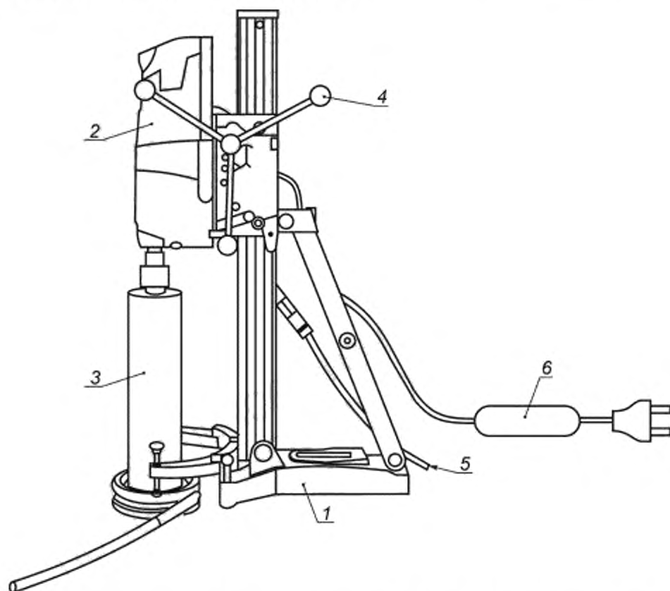
1 — сверлильная стойка; 2 — сверлильная головка; 3 — алмазная коронка; 4 — рукоятка подачи для перемещения сверлильной головки вверх и вниз; 5 — жидкостная система; 6 — УЗО (устройство защитного отключения), если поставляется
