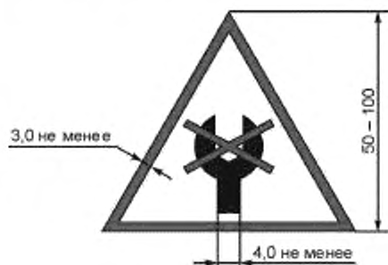
Рисунок 9 — Рекомендуемый предупреждающий знак
