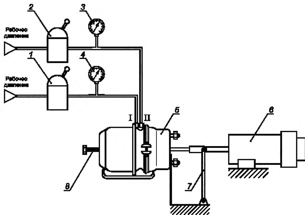
1, 2 — краны точного регулирования; 3, 4 — манометры; 5 — объект испытаний; 6 — нагрузочный цилиндр противодействия; 7 — направляющий рычаг; 8 — винт растормаживания пружинного энергоаккумулятора. I — подвод воздуха в рабочую полость, II — подвод воздуха в пружинную полость
