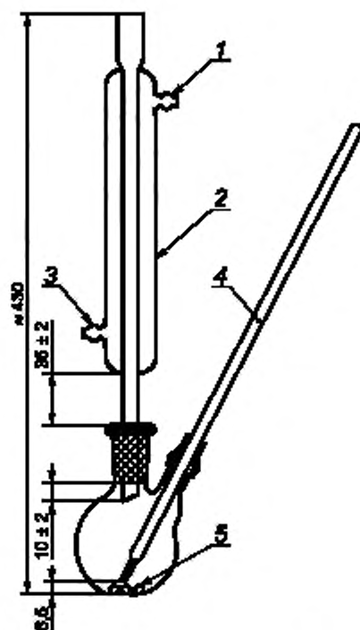
1 — выпуск воды; 2 — рубашка водяного охлаждения; 3 — впуск воды; 4 — устройство измерения температуры (экологически безопасный термометр или термопара); 5 — гранулы для предотвращения бурного кипения
