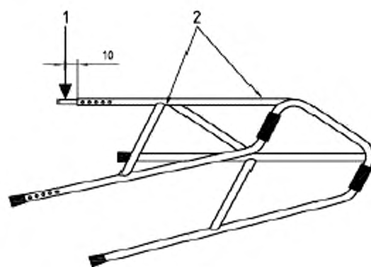
1 — нагрузка; 2 — упоры
