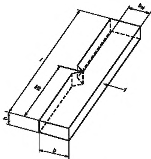
Рисунок 1 — Удар по Шарпи в ребро b образца с надрезом
