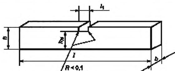
Рисунок 4 — Надрез типа А
