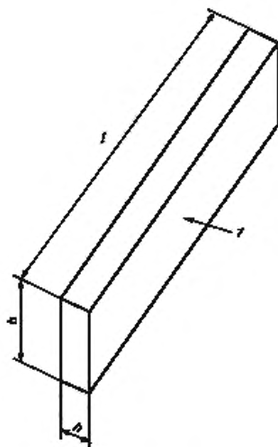
Рисунок 2 — Удар по Шарпи плашмя f
