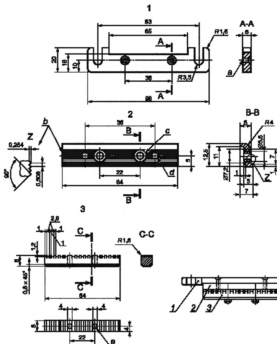
Рисунок 2 — Детали одного типа зажима, отвечающего требованиям 5.1
