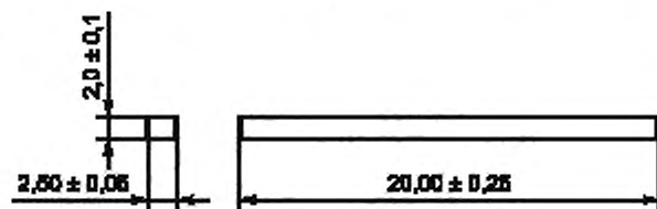
Рисунок 4 — Размеры образца для испытаний
