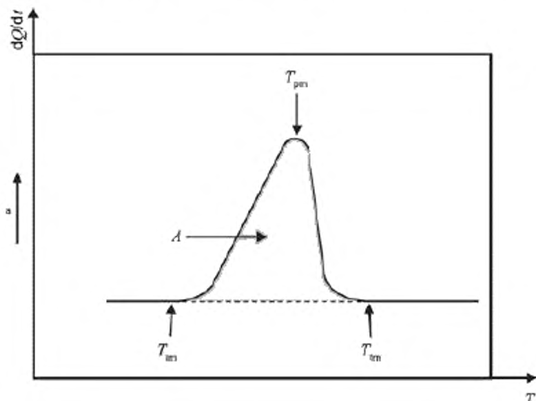
Рисунок 1 — Определение энтальпии перехода
