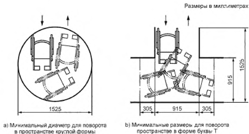
Рисунок A.4 — Пространство для поворота инвалидной коляски
