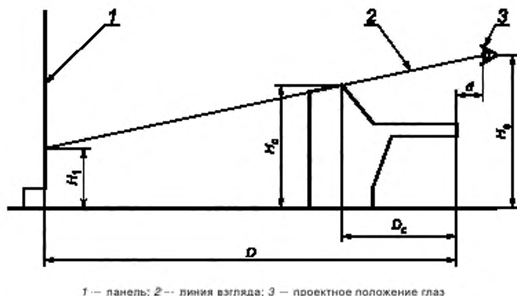
Рисунок 7 — Высота рабочей станции управления и линия взгляда поверх нее
