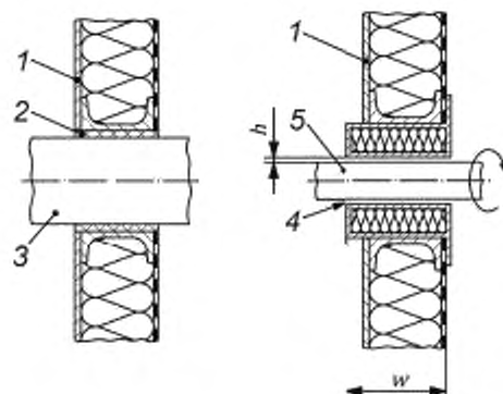
Рисунок А.14 — Пример проектирования звукоизолирующей стенки, через которую проходят трубки, оси, рукоятки и пр.
