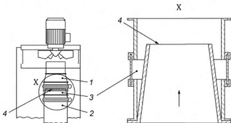
Рисунок А.6 Изолированное соединение транспортировочного вентилятора и воздухопроводов
