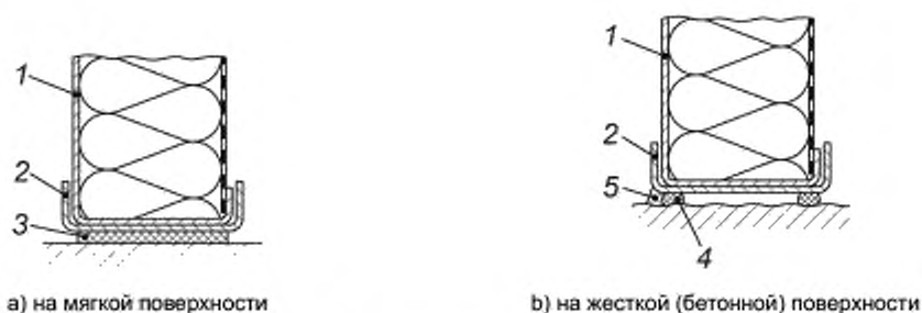
Рисунок А.12 — Пример установки стенки кожуха
