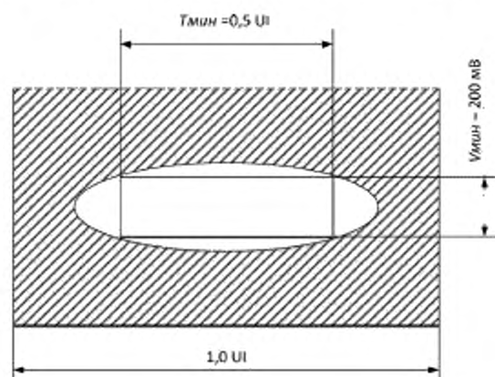
Рисунок 4 — Глаз-диаграмма
