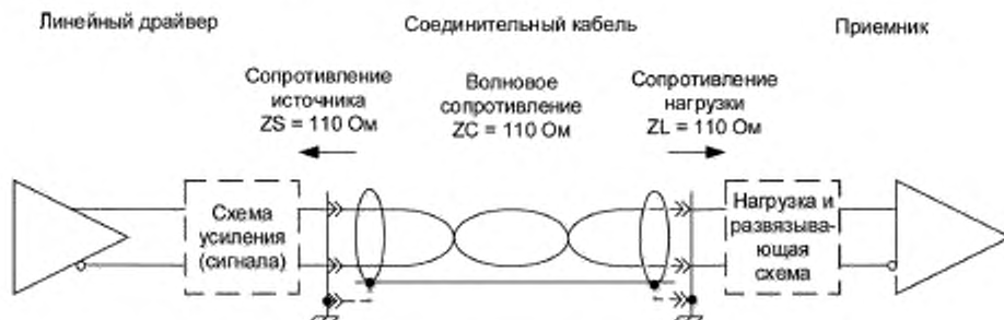
Рисунок 1, лист 1 — Упрощенный пример конфигурации сети (симметричной)
