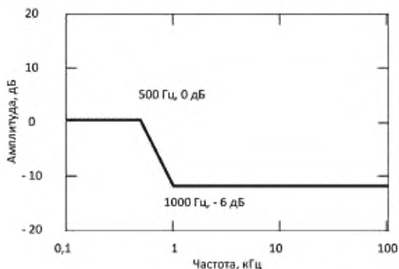
Рисунок 3 — Маска подавления фазового дрожания (обязательной не является)
