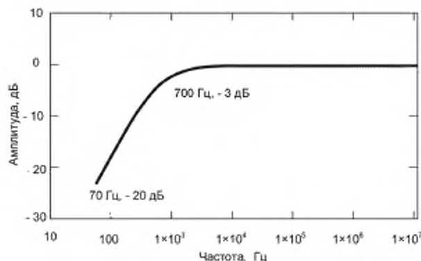
Рисунок 2 — Фильтр для измерения собственного фазового дрожания
