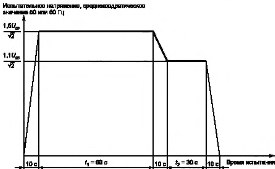
Рисунок 1 — Испытание на частичный разряд; напряжение в зависимости от времени
