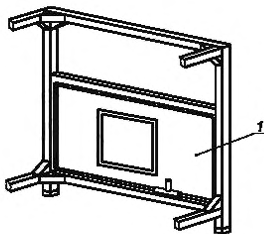
б) Вид на монтажную панель изнутри камеры
