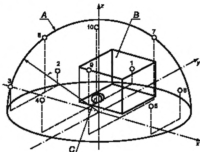
1, 2, 3, 4, 5, 6, 7, 8, 9, 10 — положения микрофона; А — измерительная поверхность; В — испытательная камера; С — место установки испытуемого вентилятора; r — радиус полусферы
