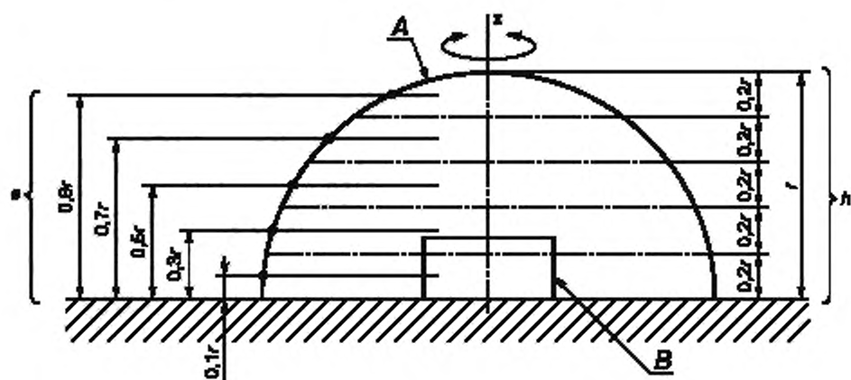
А — измерительная поверхность; В — испытательная камера; e — вертикальная проекция траектории микрофона; h — высота соответствующих областей полусферы; r — радиус полусферы; z — ось вращения механизма сканирования микрофона
