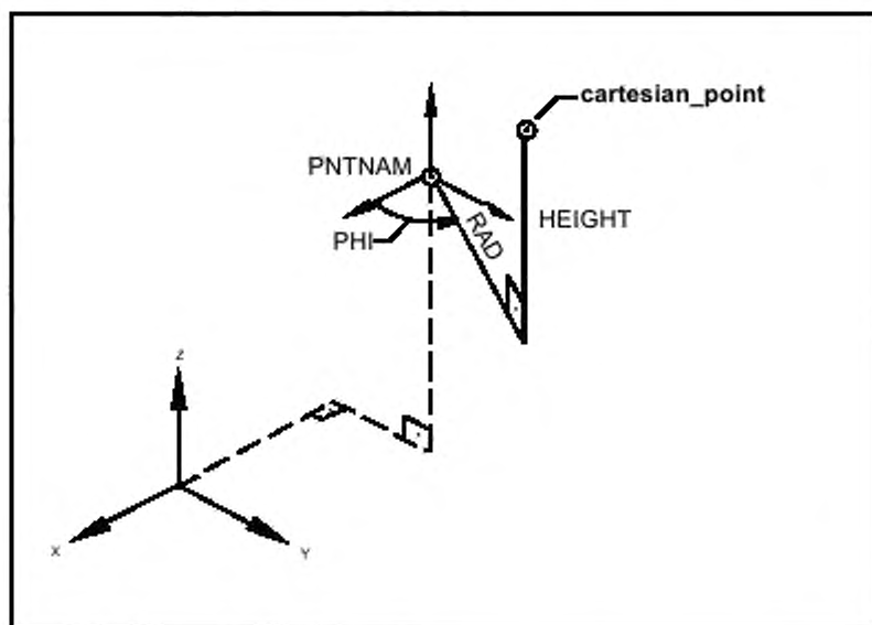
Cartesian_point — новая декартова точка; PNTNAM — исходная декартова точка; RAD — цилиндрическая координата (радиус); HEIGHT — цилиндрическая координата (высота); PHI — цилиндрическая координата (угол «фи»)
