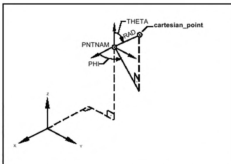
Рисунок A.10 — Функция Pnt_Polar_Relative
