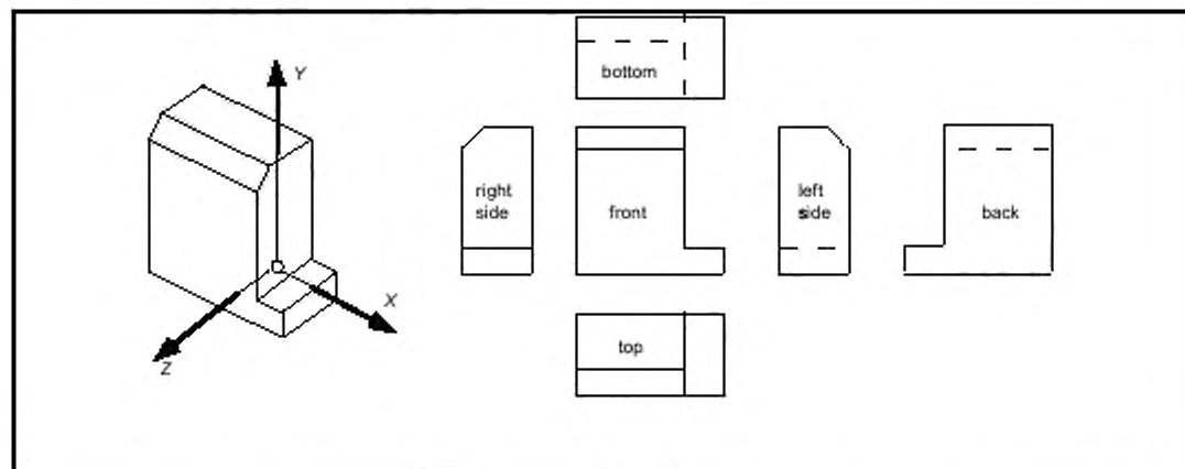
Bottom — вид снизу; right side — вид справа; left side — вид слева; front — вид спереди; back — вид сзади; top — вид сверху
