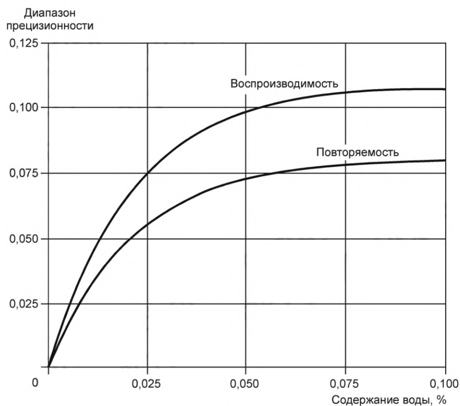
Рисунок 2 — Прецизионность метода определения воды в нефти
