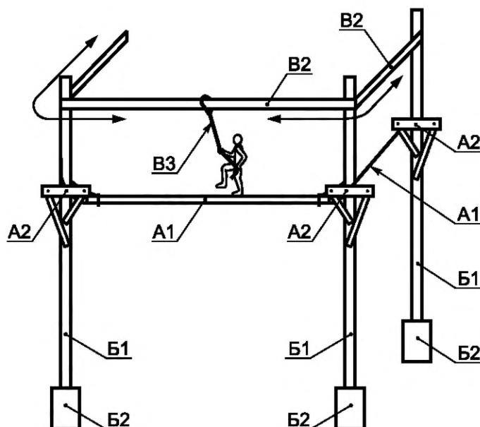
А — рабочие системы: А1 — элементы, А2 — платформы; Б — опорные системы: Б1 — опоры (чурбаки, булжники, иные опорные конструкции), Б2 — фундаменты, анкеры; В — страховочные линии: В2 — непрерывная страховочная линия, В3 — самостраховка
