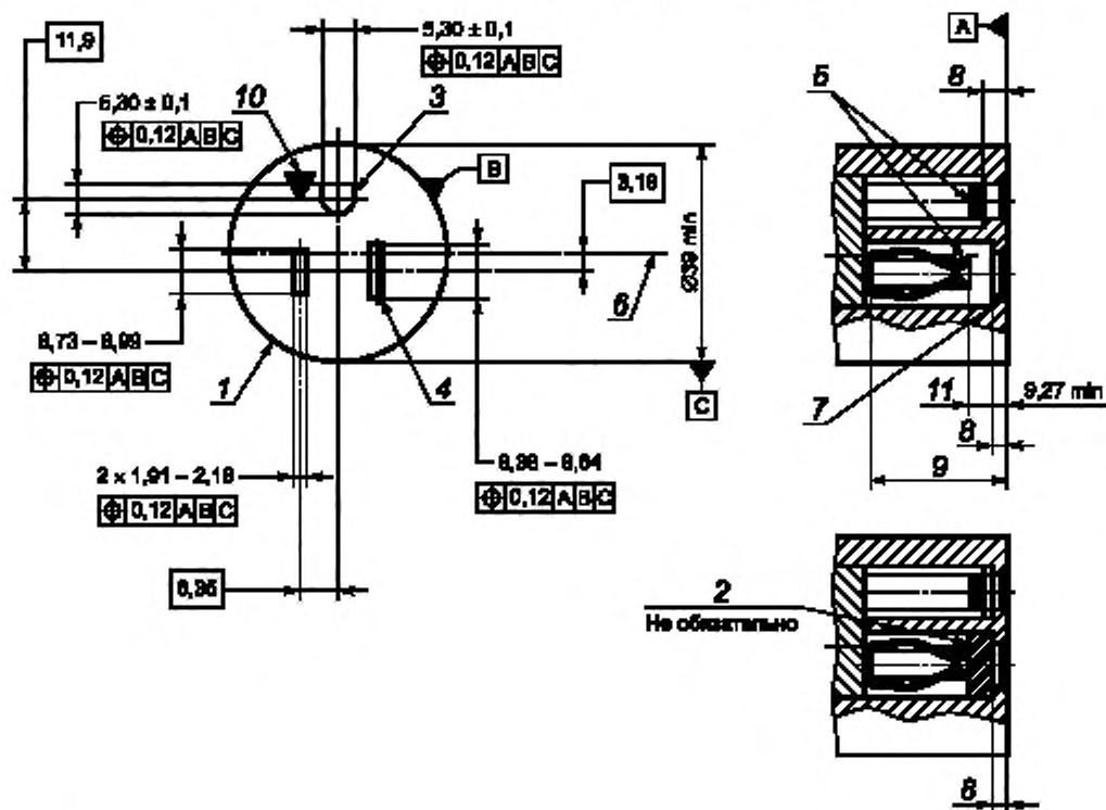
Стандартный лист 1 Двухполюсная штепсельная розетка с заземляющим гнездом на переменный ток 15 А и напряжение 125 В
