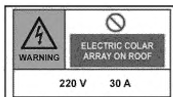
Рисунок F.5 — Пример знака, располагаемого на выключателе — разъединителе ФБ (главном выключателе ФБ), и идентичный знак МЭК
