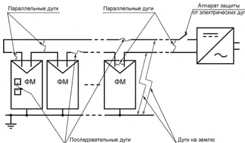
Рисунок 9 — Примеры дуг различного типа
