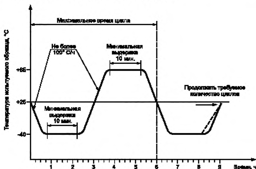
Рисунок 4 — Профиль изменения температуры при термоциклировании
