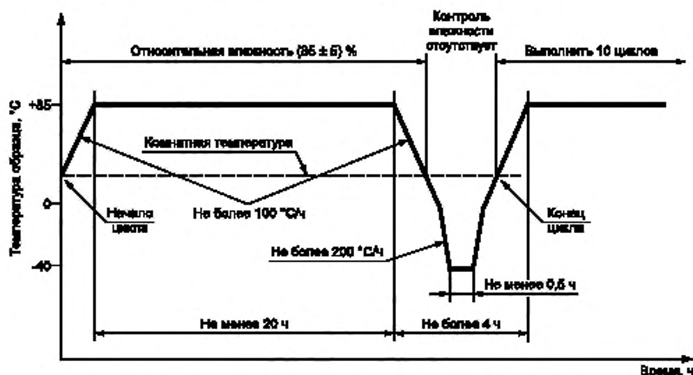
Рисунок 5 — Цикл термоциклирования при высокой влажности
