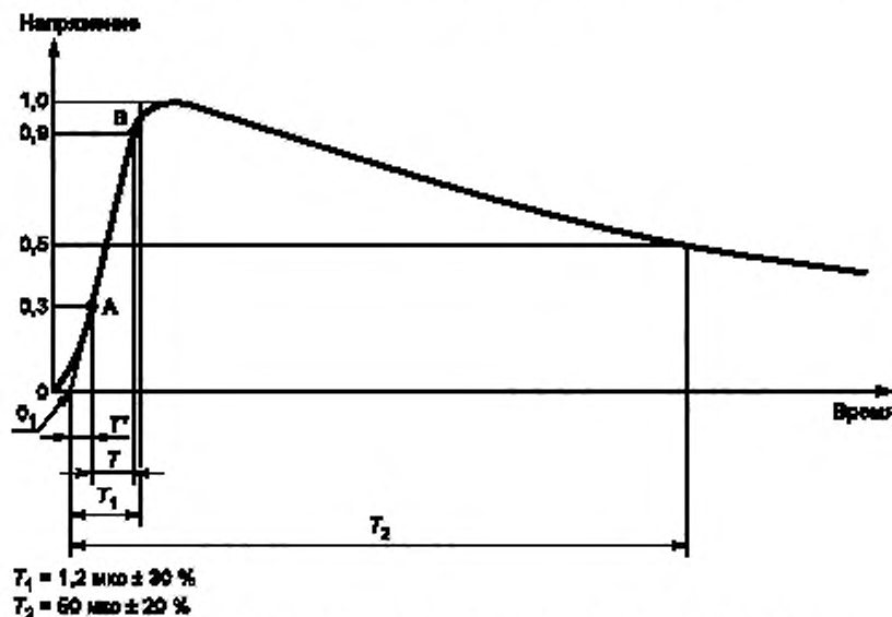
Рисунок 7 — Форма импульса испытательного напряжения 1,2/50
