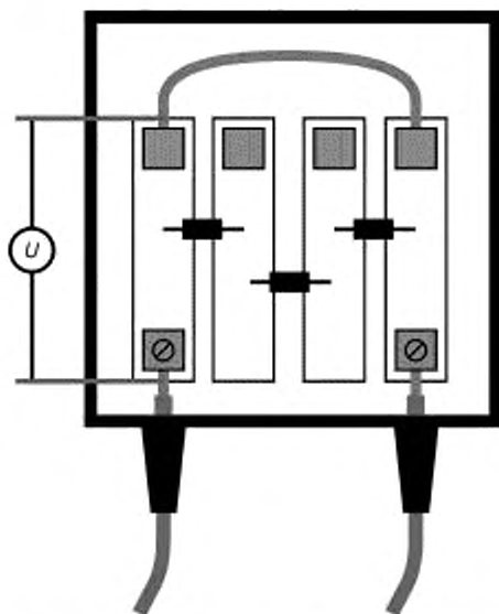
Рисунок 6 — Пример измерения напряжения для определения сопротивления контактов
