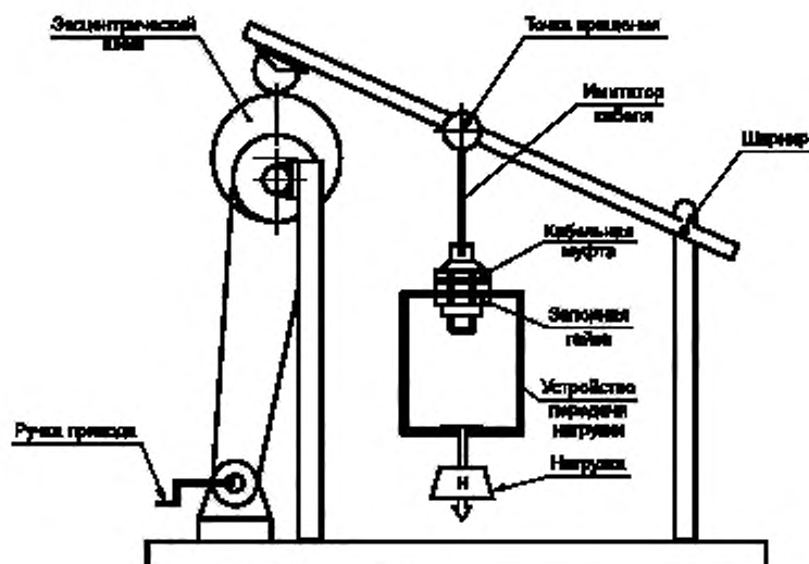
Рисунок 2 — Типичная установка для испытания надежности закрепления кабеля (провода) натяжением
