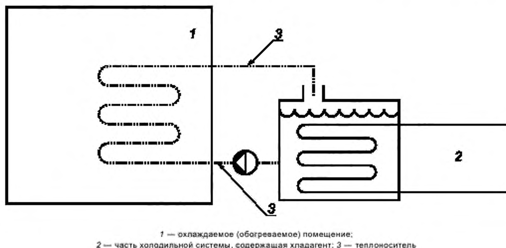
Рисунок 6 — Промежуточная система с открытым уровнем
