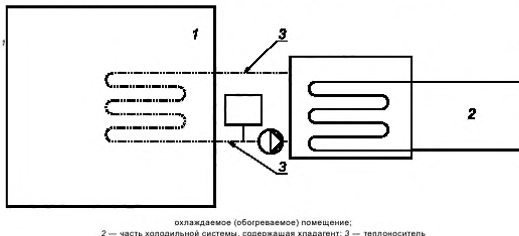
Рисунок 5 — Закрытая промежуточная система
