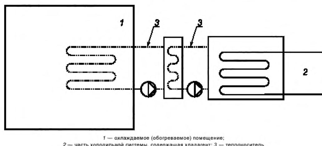
Рисунок 8 — Промежуточная сдвоенная система
