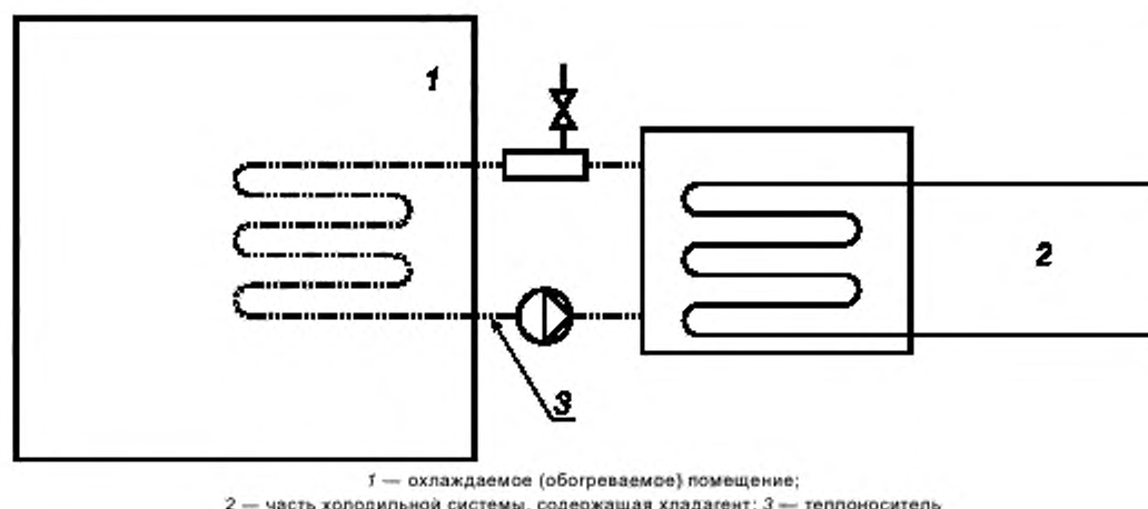
Рисунок 7 — Закрытая промежуточная система с вытяжкой
