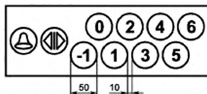
Рисунок F.3 — Пример двухрядного исполнения устройства управления с круглыми кнопками
