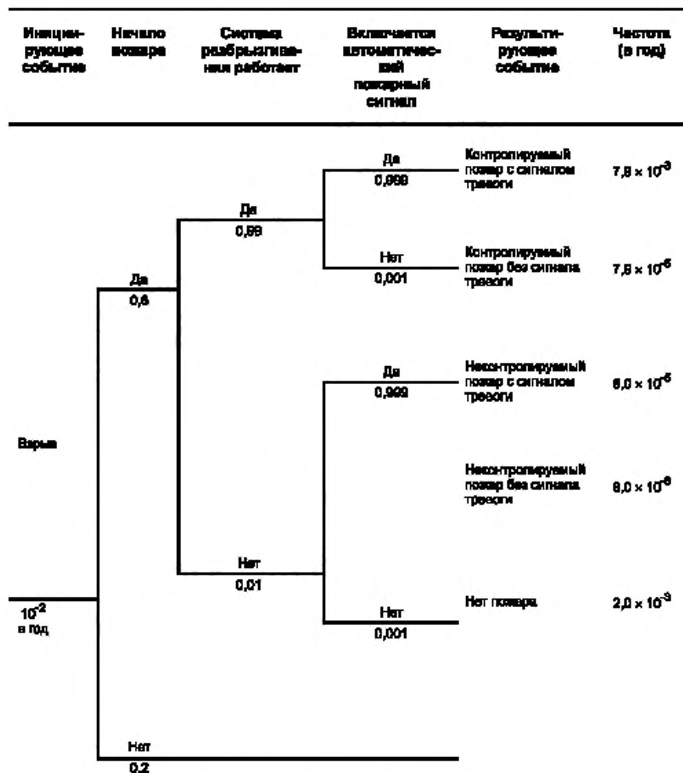
Рисунок А.3 — Пример «дерева событий» для взрыва пыли
