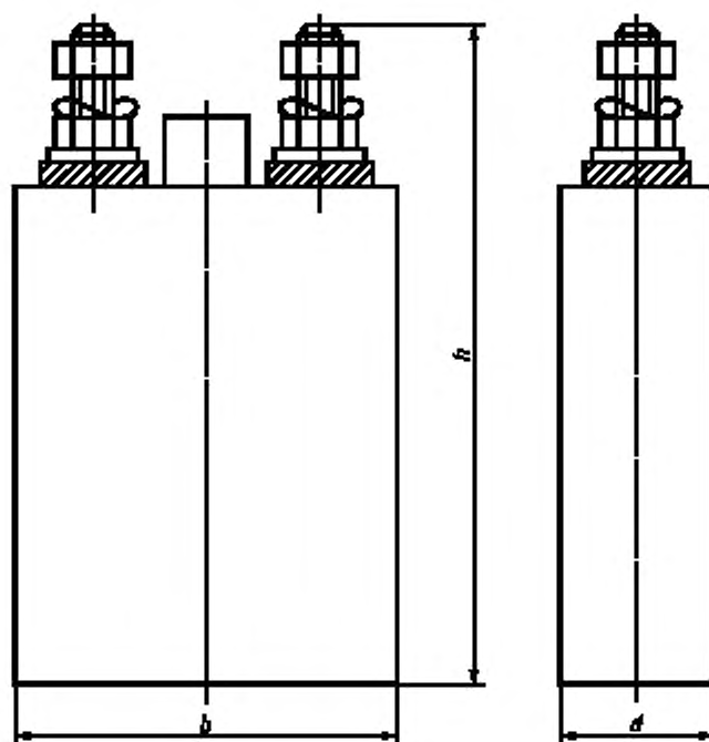
Рисунок 1 — Пример герметичного призматического аккумулятора
