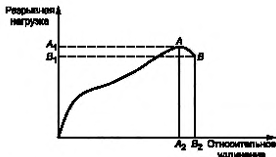
Рисунок 1 — Типичная кривая разрывная нагрузка — относительное удлинение
