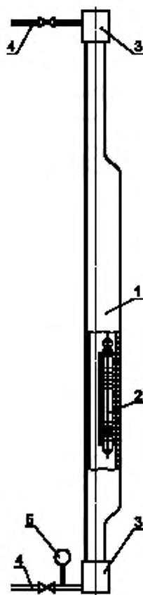
1 — скважинная камера; 2 — пробка, 3 — переходник со штуцерами; 4 — трубопроводы с залорной арматурой; 5 — манометр
