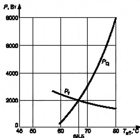
Рисунок А.1
