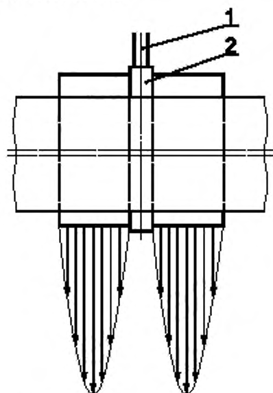
1 — смазочное отверстие; 2 — смазочная канавка
