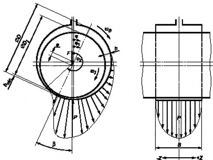
Рисунок 2 — Иллюстрация обозначений
