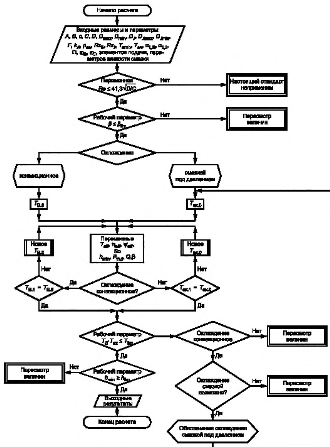
Рисунок 1 — Схема расчета
