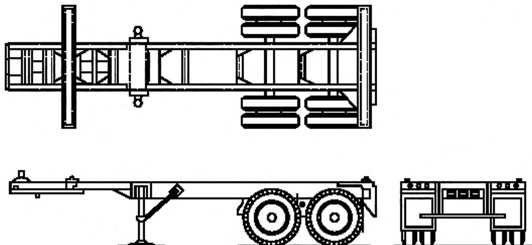
Рисунок В.1 — Типовое шасси с четырьмя поворотными замками
