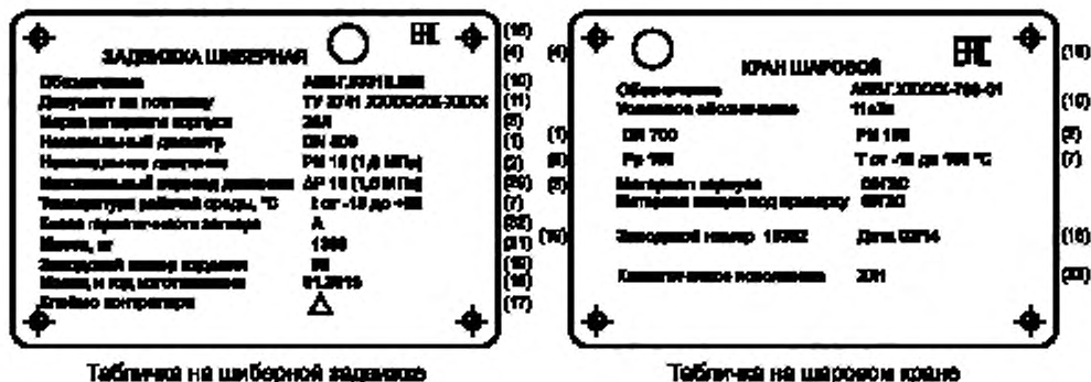
Табличка на шиберной задавке
