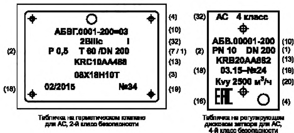
Рисунок Г.5 — Примеры расположения маркировки на табличке
