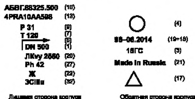
Рисунок Г.3 — Пример расположения маркировки на корпусе углового регулирующего клапана
