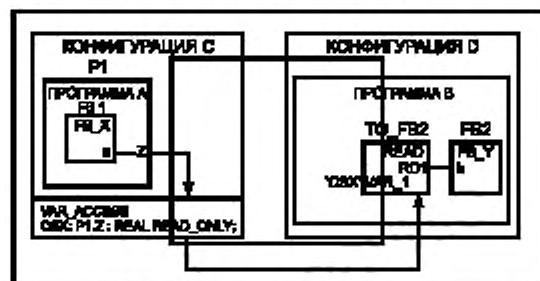
г) Взаимодействие через пути доступа
