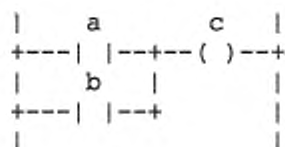
a) «Монтажное ИЛИ» в языке LD
