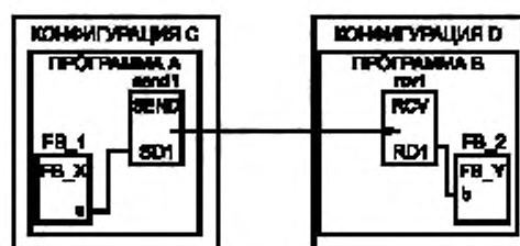
в) Функциональные блоки взаимодействия
