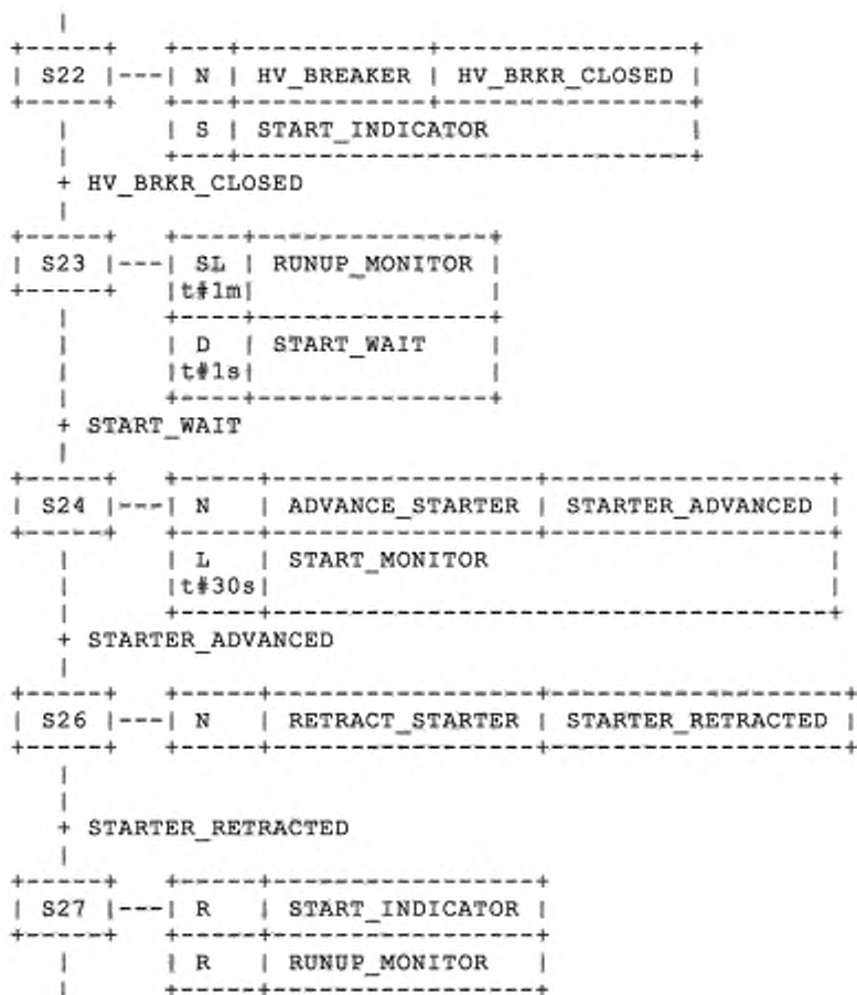
а) Представление SFC
