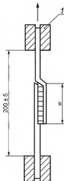
1 — зажим, w — ширина сварного (клевого) соединения
