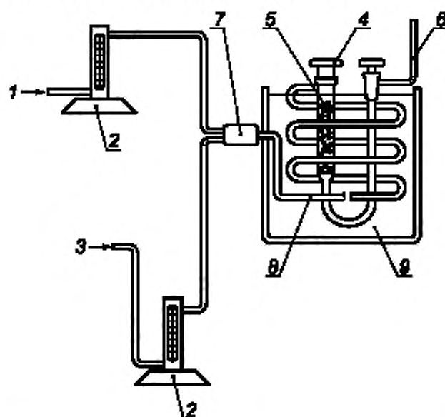
1 — n-бутан; 2 — расходомер; 3 — сухой воздух без органических примесей; 4 — трубка для пробы; 5 — активированный уголь; 6 — вытяжной вентилятор; 7 — двухходовой кран; 8 — змеевик для нагрева газа длиной 1,9 м; 9 — водяная баня
