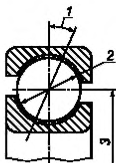
1 — угол контакта; 2 — диаметр шарика D_{\text{ball}} ; 3 — диаметр окружности центров шариков D_{\text{pit}}
