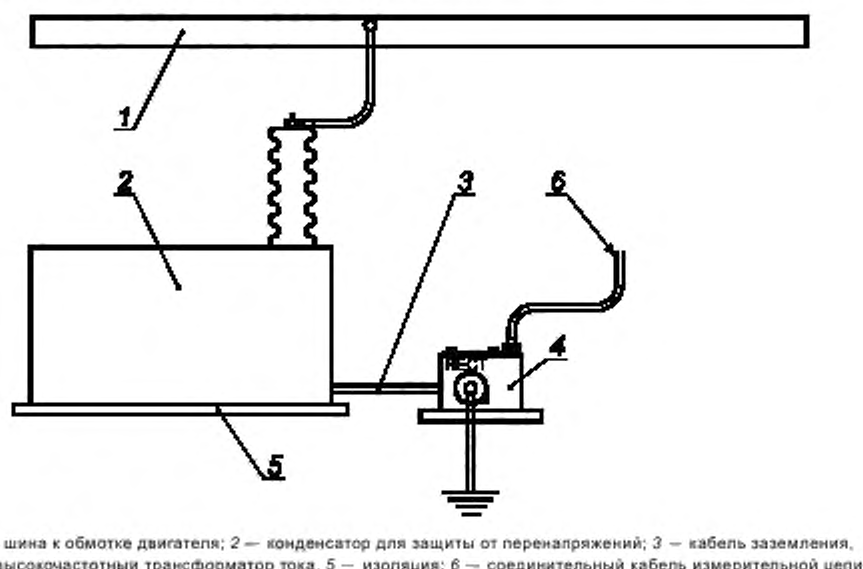
Рисунок 8 — Схема установки высокочастотного трансформатора тока на кабеле от конденсатора для защиты обмотки статора от перенапряжений
