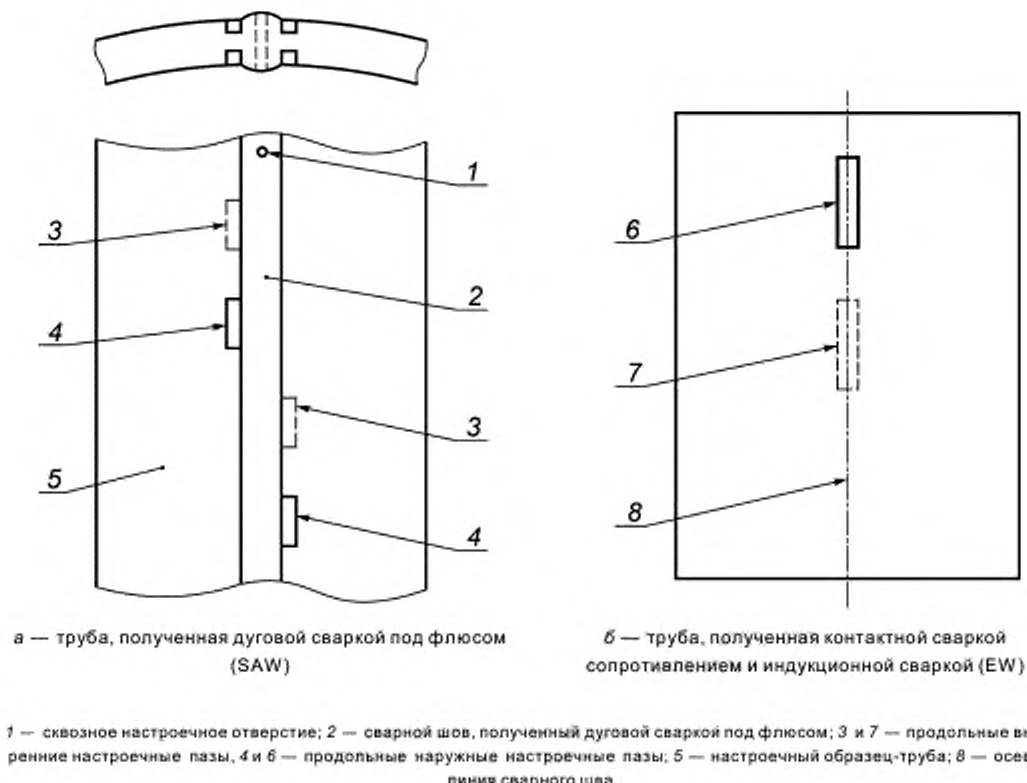
Рисунок 1 — Схема настроечного образца-трубы
