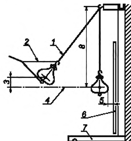
1 — трос; 2 — узелка для подъема мешка; 3 — высота падения мешка; 4 — центр мешка в состоянии покоя; 5 — расстояние между образцом и мешком, висющим в свободном состоянии; 6 — образец, закрепленный в раме; 7 — опора; 8 — высота подвеса
