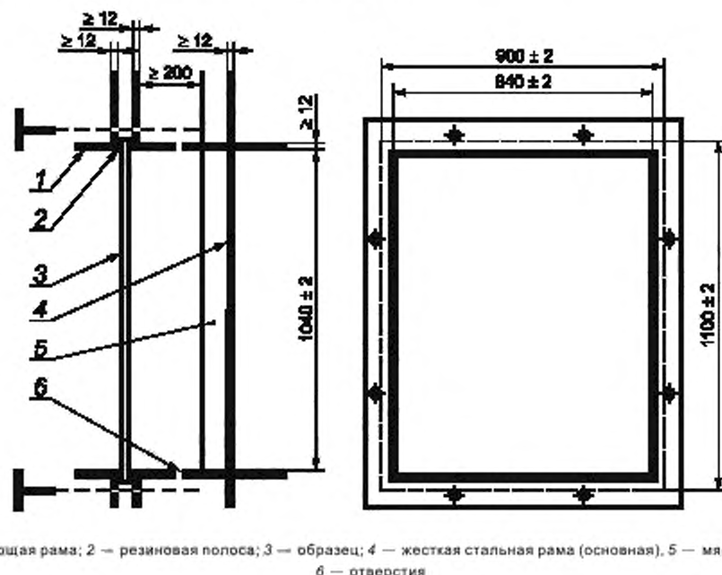
Рисунок 1 — Оборудование для крепления образца
