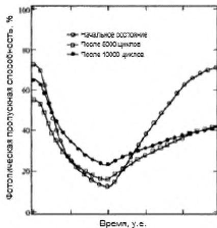
Рисунок 5 — Фотохимическая пропускная способность как функция времени, измеренного на различных этапах циклических испытаний типового окна с ЭХП
