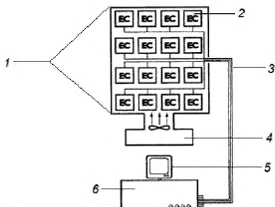
1 — плоскость испытания 1220 × 1830 мм; 2 — стекла с ЭХП; 3 — электрические выводы и кабели термпар; 4 — термощаф; 5 — компьютер; 6 — многоканальная цифровая автоматизированная система управления и сбора данных
