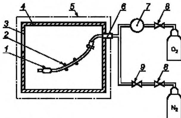
1 — тестируемая трахеальная трубка; 2 — опора трахеальной трубки с использованием двух хомутов; 3 — отверстие для доступа пучка лазерного излучения; 4 — защитный корпус (вид сбоку); 5 — крышка корпуса (может состоять из множества элементов); 6 — стопор обратного выброса; 7 — измеритель расхода кислорода и регулятор; 8 — регулятор давления с входными и выходными датчиками; 9 — быстродействующий клапан для инертного газа
