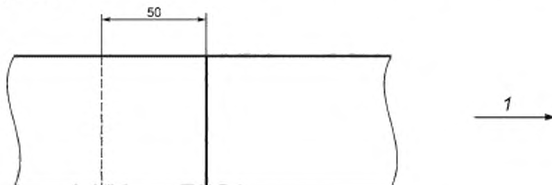
Рисунок Г.2 — Поперечные стыки матов
