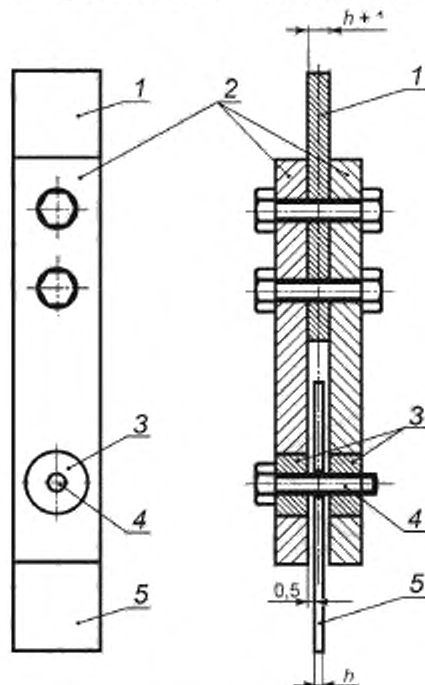
1 — распорная плита (толщина = h + 1 мм); 2 — боковая плита из закаленной стали; 3 — втулки из закаленной стали, посадка скользящая в боковых плитах (опционально); 4 — гладкий штифт; 5 — образец для испытаний
