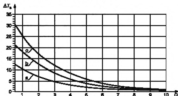
Рисунок 3 — Повышение температуры поверхности в области разброса порога возникновения ожога, приведенного на рисунке 2 для металлов, покрытых лаком толщиной в 50, 100 и 150 мкм
