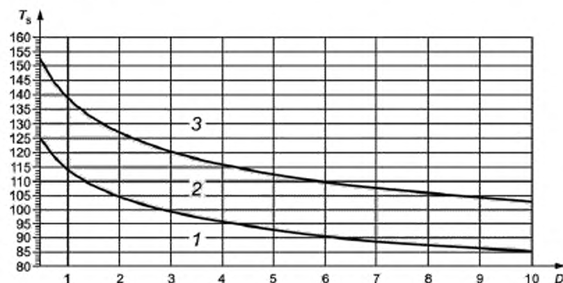
Рисунок 7 — Область разброса порога возникновения ожога, когда кожа находится в контакте с горячей гладкой поверхностью из древесины
