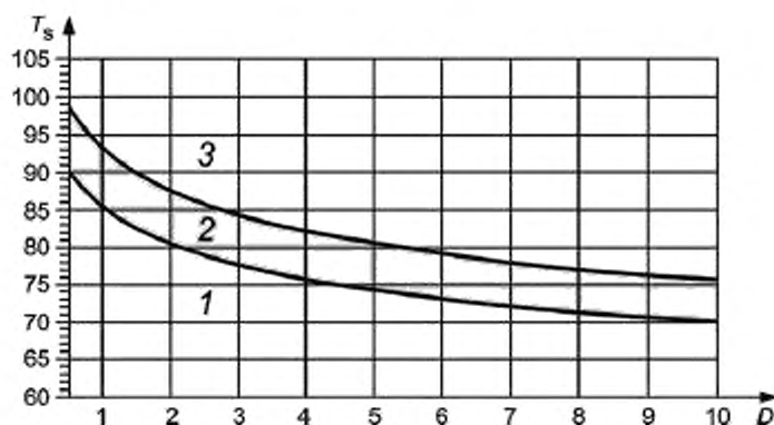
Рисунок 6 — Область разброса порога возникновения ожога при контакте кожи с горячей гладкой поверхностью из пластмассы
