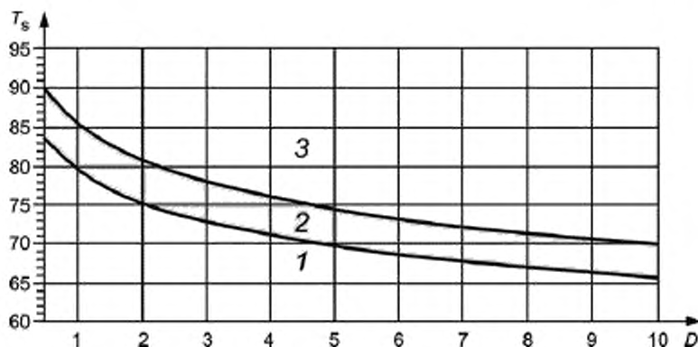
Рисунок 5 — Область разброса порога возникновения ожога, когда кожа находится в контакте с горячей гладкой поверхностью, выполненной из керамики, стекла и камня
